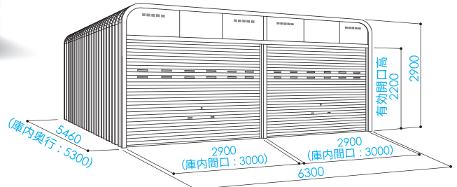
(単位: mm) ※寸法図は54CB型2連棟です。
