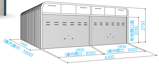
(単位: mm) ※寸法図は54CR型2連棟です。
