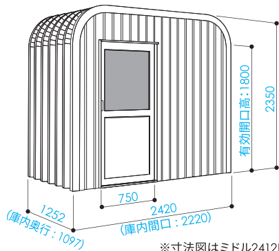
※寸法図はモデル2412H型です。
