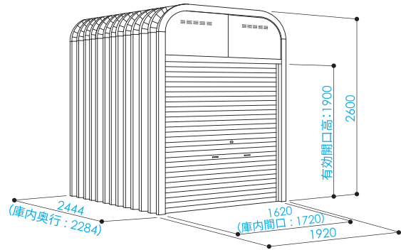
(単位: mm) ※寸法図はイグルーミニ24です。
