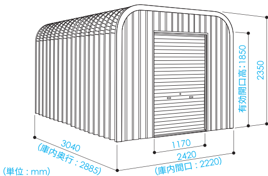
※寸法図はモデル2430S型です。
