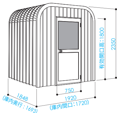
※寸法図はミニ1918D型です。
