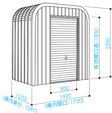
※寸法図はミニ1912S型です。
